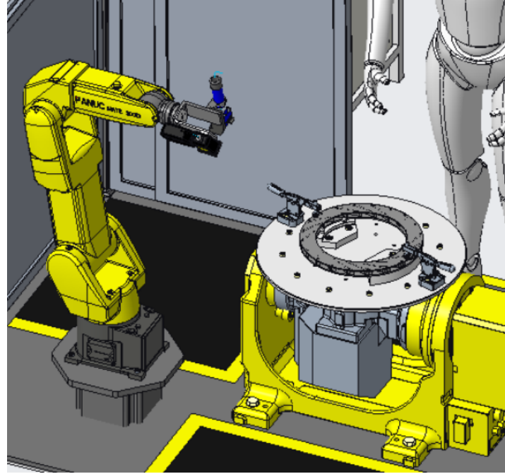
Simulace robotizovaného pájecího pracoviště
